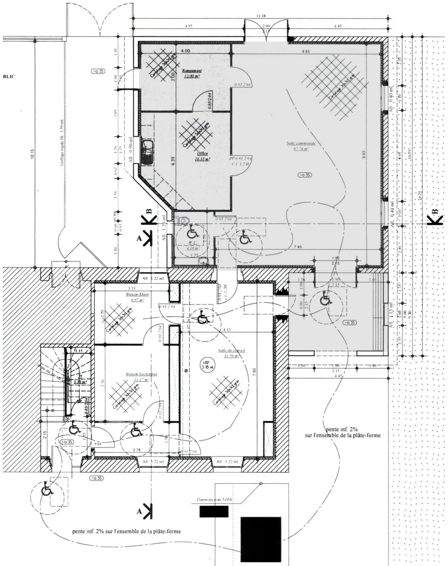
Plan du rez-de-chaussée En gris clair : tranche n°2
